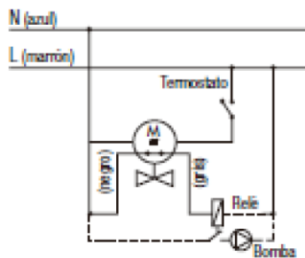
NA 4 cables
